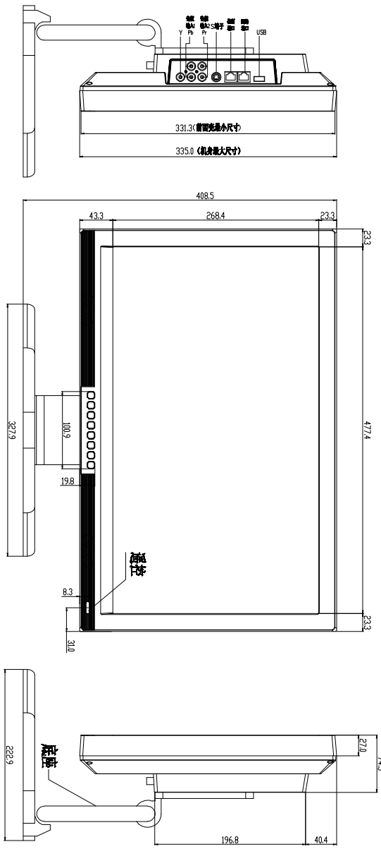
左侧视图
