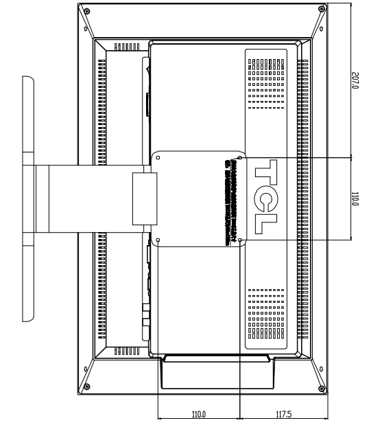
后视图
