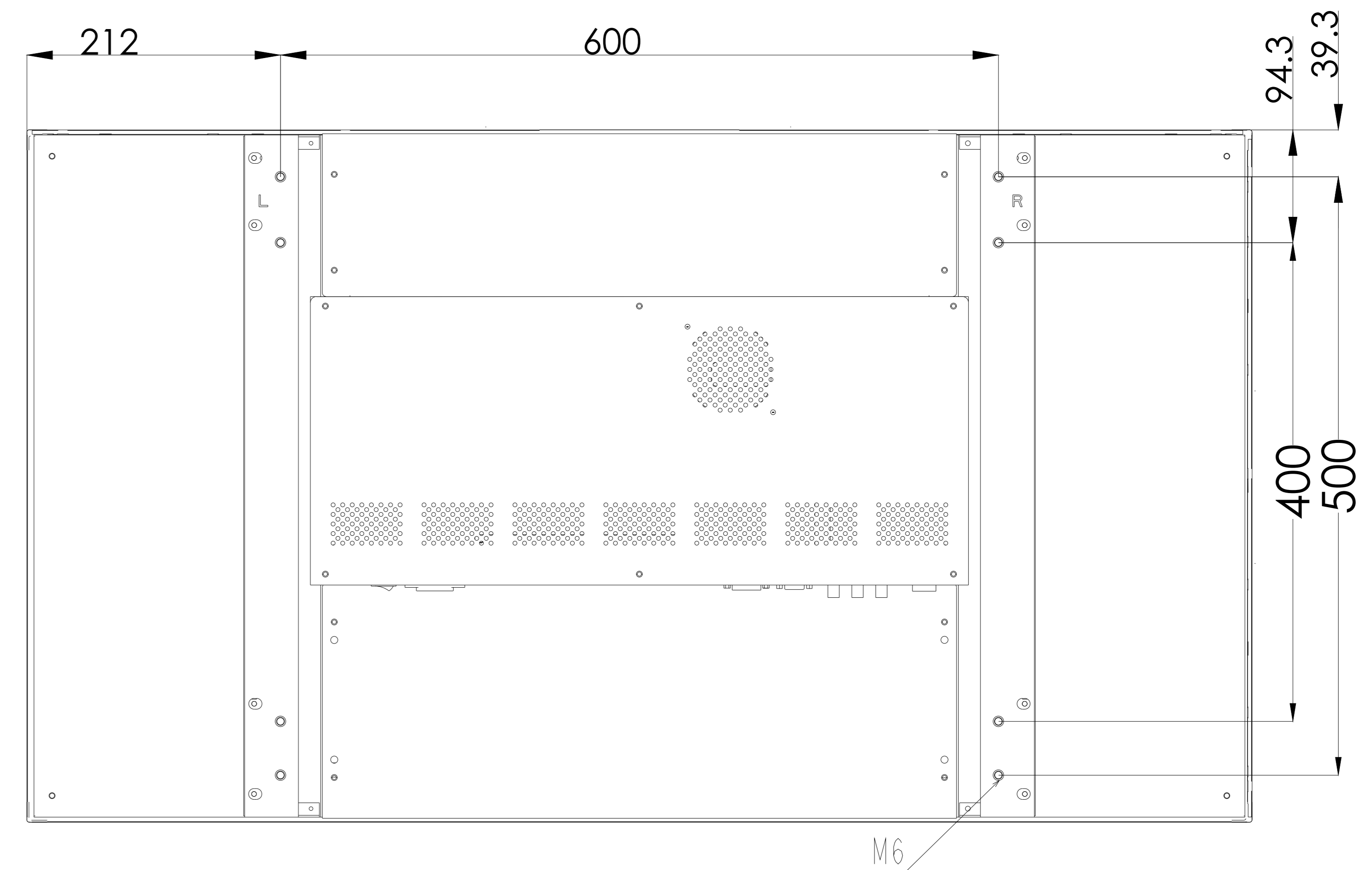
后视图
