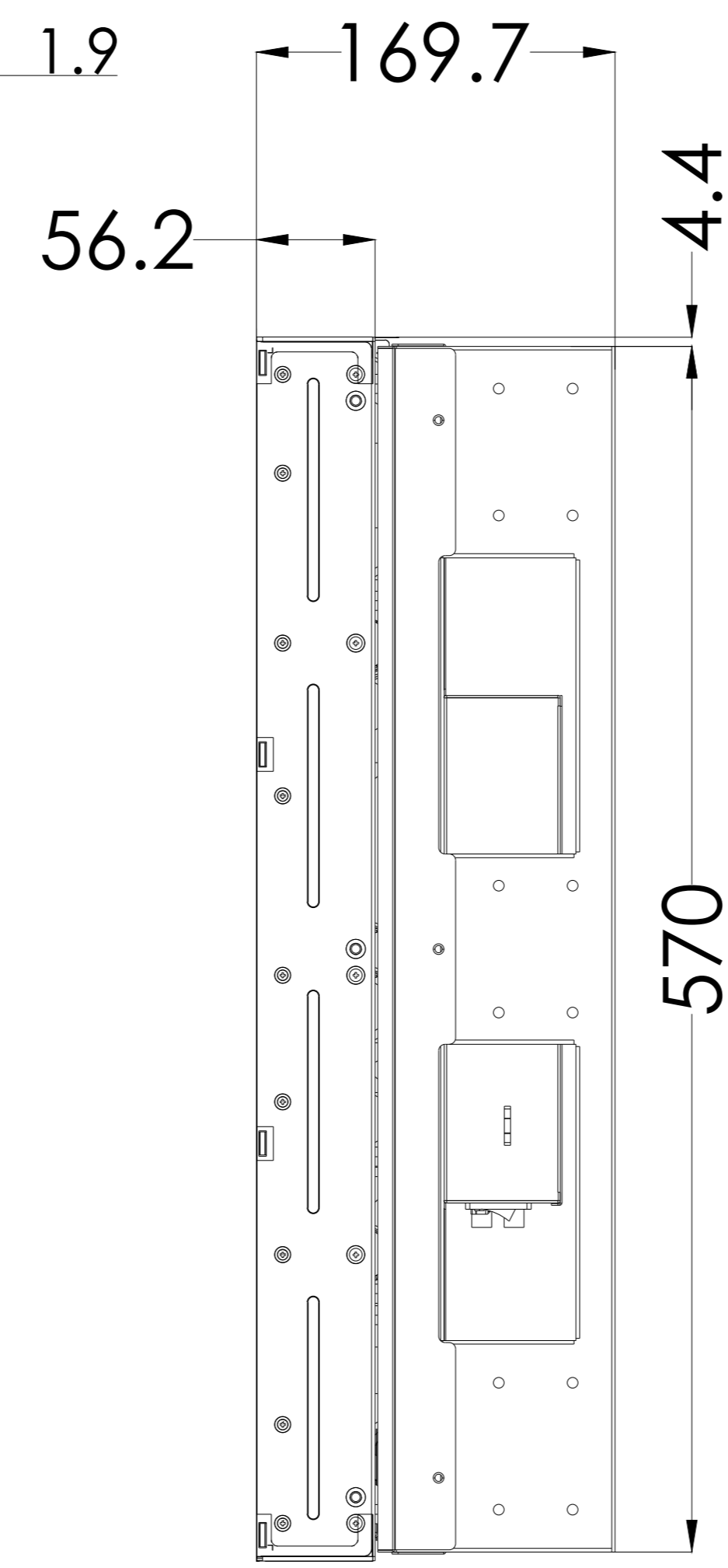
侧视图
