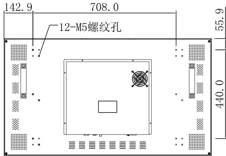
后视图
