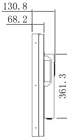
侧视图
